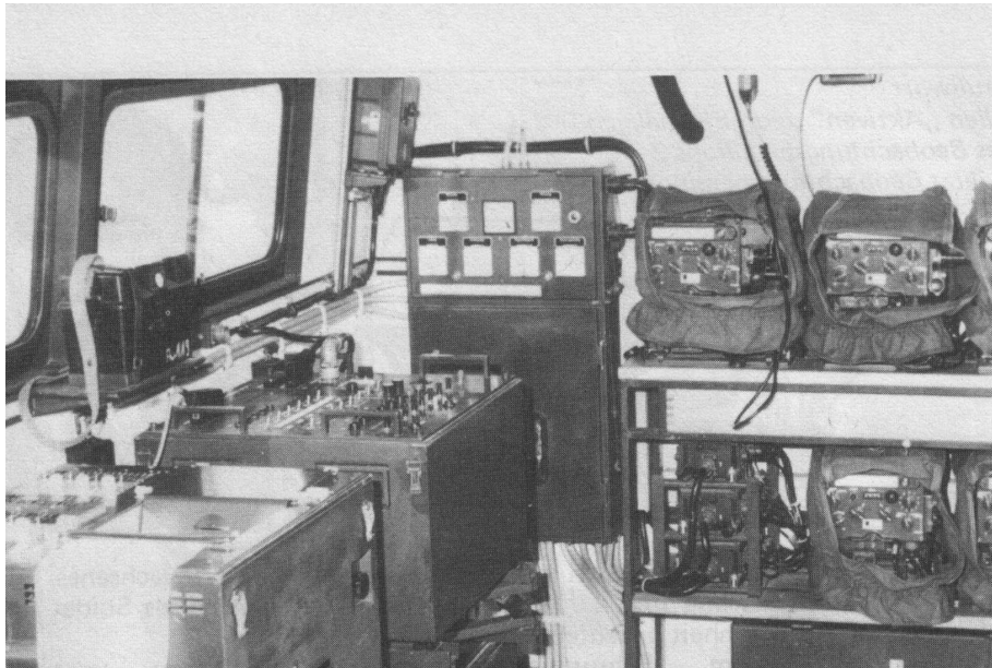
Blick in das Innere des Schallmessaufnahme Kfz.
